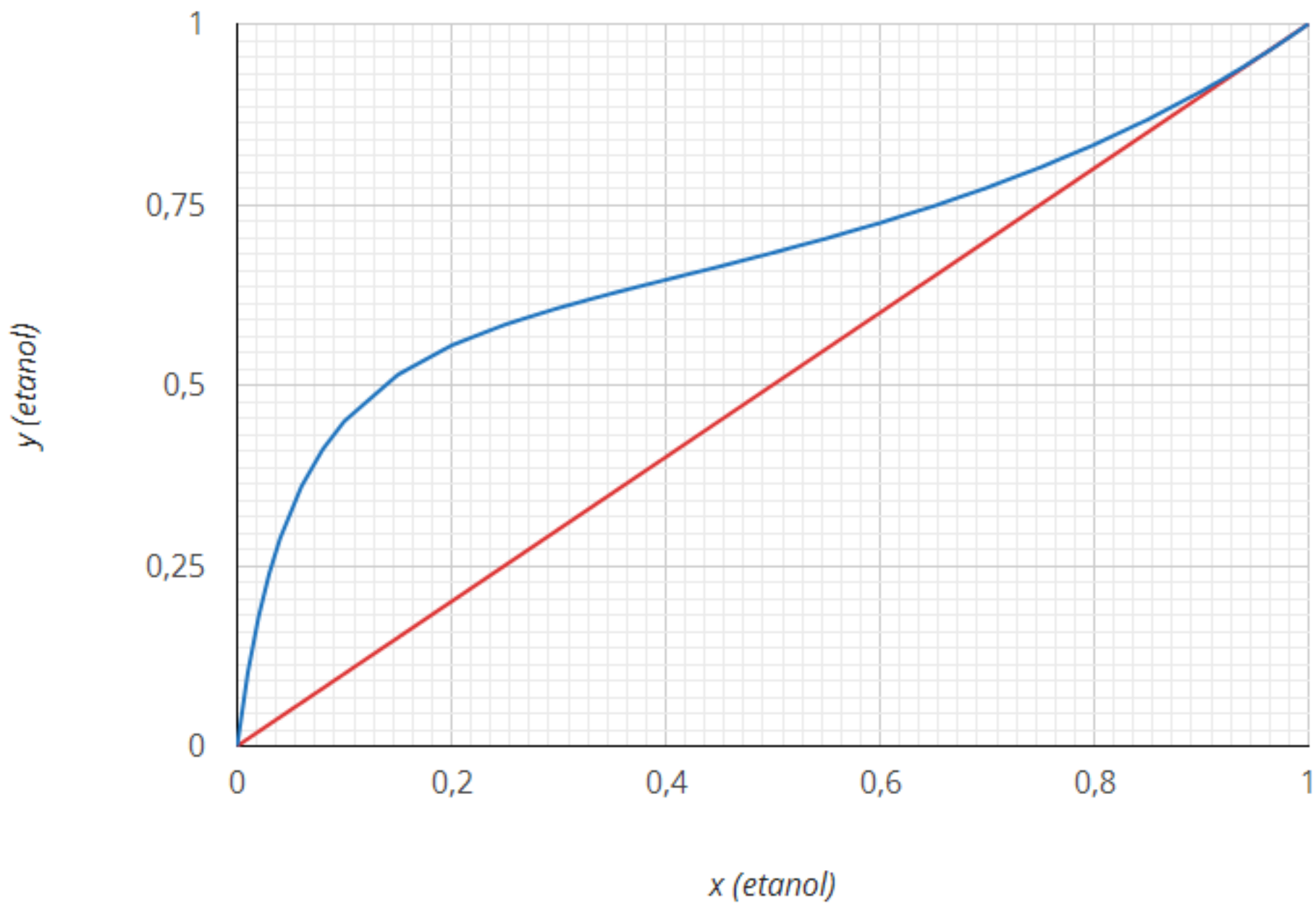
Wykres równowagowy układu woda-etanol
